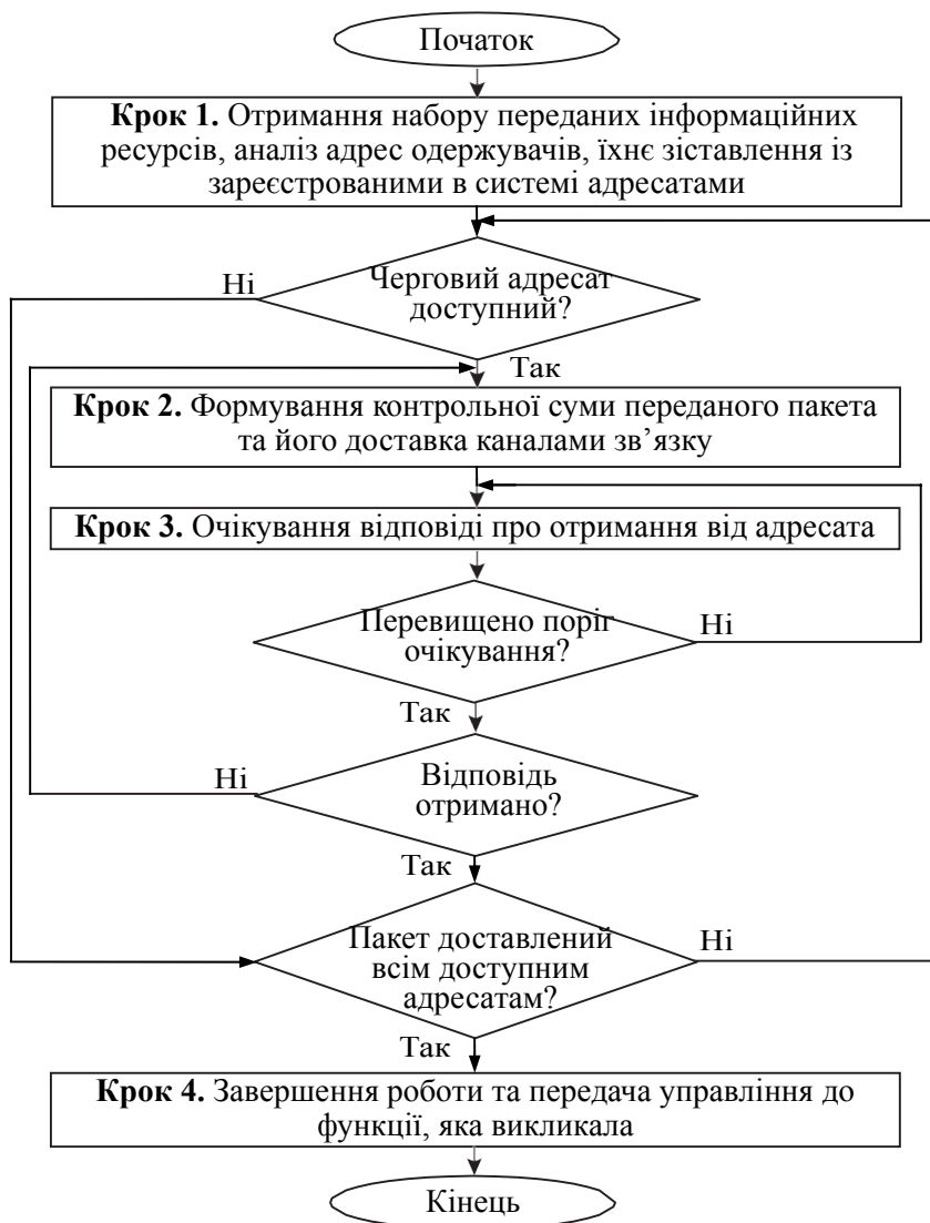
Рис. 3. Схема алгоритму роботи функції інформаційної взаємодії вузлів розподіленої АС
