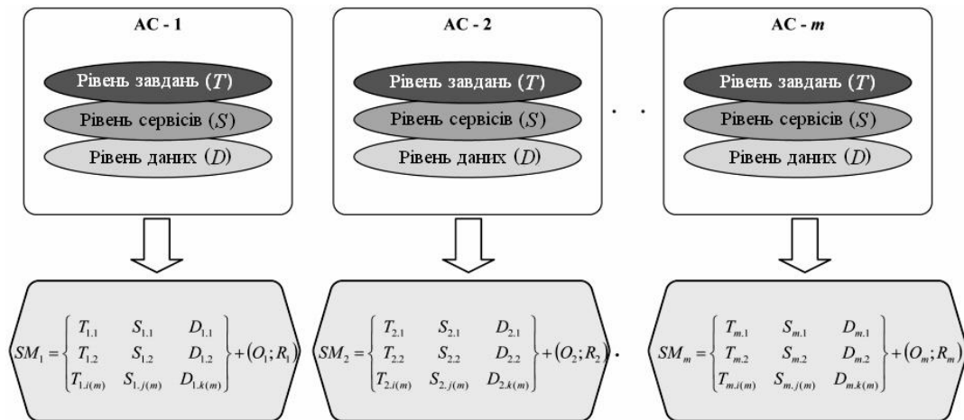
Рис. 2. Семантична модель взаємодії різнорідних АС
